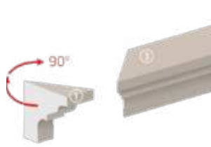
3_SPAJANJE FASADNE LAJSNE
