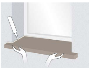
6_LEPLJENJE KLUPICE NA PODLOGU I ZAPTIVANJE MONTAŽNOM GIT MASOM
