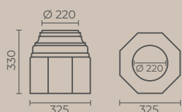
STOPA - HS 22F
