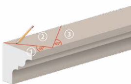
1_OBELEŽAVANJE LINIJE SEČENJA
